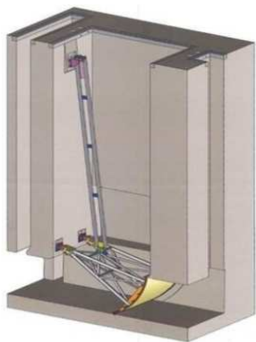
Vue d'ensemble d'une vanne aqueduc (une vanne aqueduc côté mer, une autre côté bassin)
